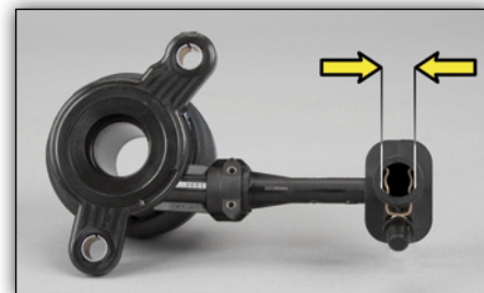
Fig. 2: LuK CSC 510 0097 10 Conexión hidráulica 13,3 mm
