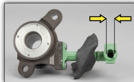
Fig. 4: LuK CSC 510 0137 10 Conexión hidráulica 12,2 mm
