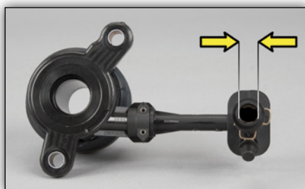
Fig. 3: LuK CSC 510 0098 10 Conexión hidráulica 11,7 mm
