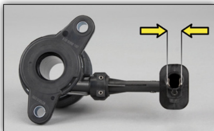
Fig. 1: LuK CSC 510 0090 10 Conexión hidráulica 12,2 mm
